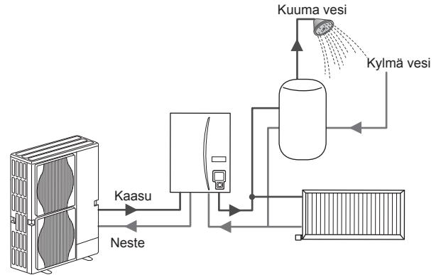
Hydroboxin kaavioesitys
